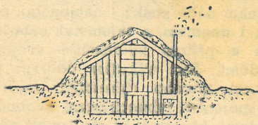
Průřez příčný
