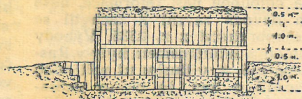
Průřez podélný
